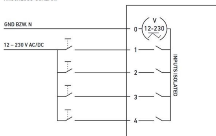
ANSCHLUSS-SCHEMA:
