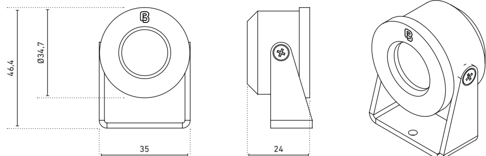
TECHNISCHE ZEICHNUNG | TECHNICAL DRAWING
