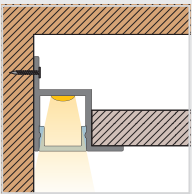
Wandmontage mit Schraube wall mounting with screw
