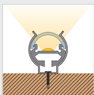
Montage mit Halteklammer mounting with clips
